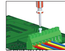
Зачистка → Гнездо № → Обжимной носик → Винтовой замок / Зачистка → Гнездо № → Винтовой замок
