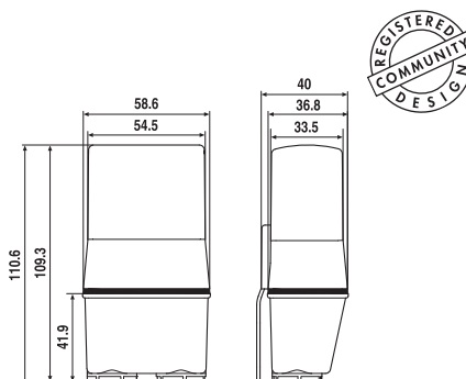
Тип 10.41
