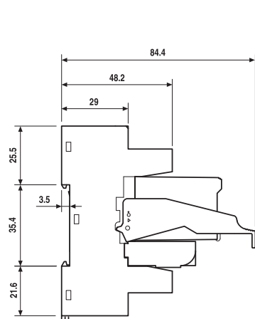
96.02 + 56.32 + 094.91.3 + 86.30
