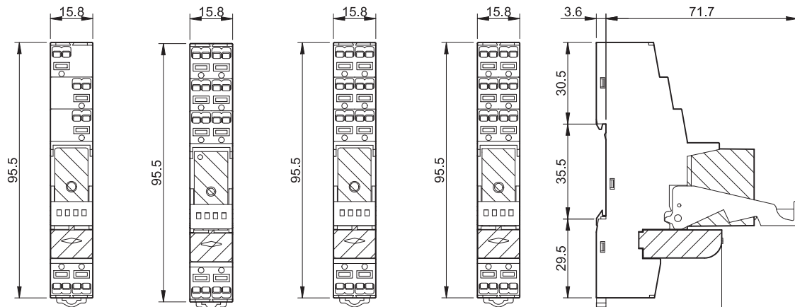
48.P3 48.P5 48.P6 48.P8 Пружинный зажим
