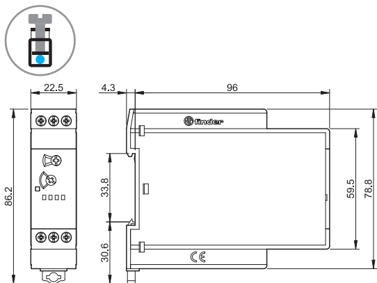
83.82 Винтовые клеммы
