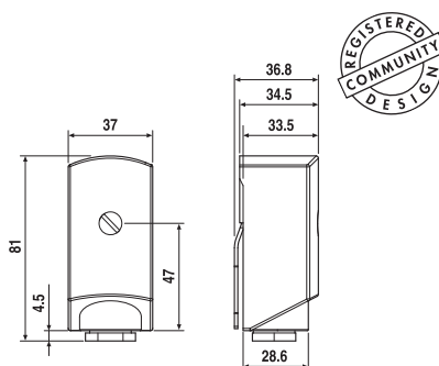
Тип 10.51
