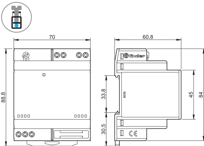
78.51 / 78.61 Винтовые клеммы
