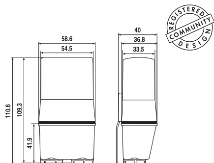
Тип 10.32
