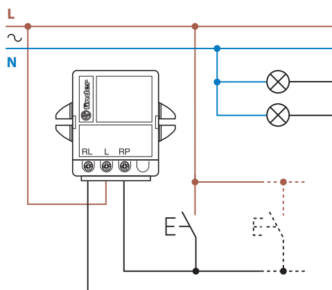
Тип 15.51 - 4-проводное соединение
