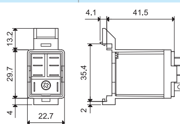
056.27 с реле
