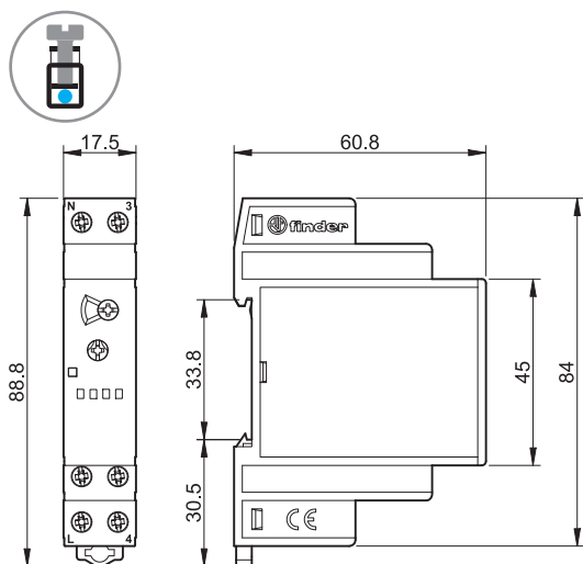
14.01 Винтовые клеммы
