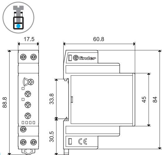
70.11 Винтовые клеммы
