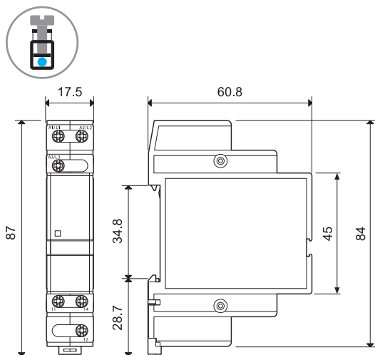
70.61 Винтовые клеммы
