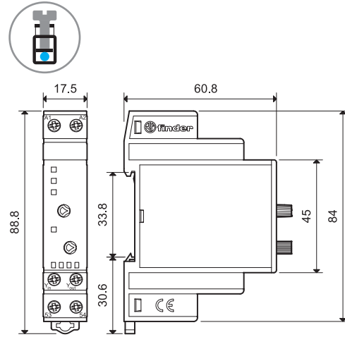
Тип 19.50
