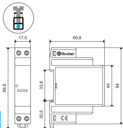
77.01 Винтовые клеммы
