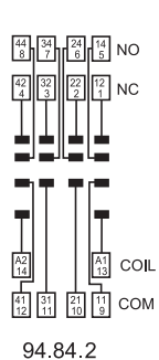
94.84.2
