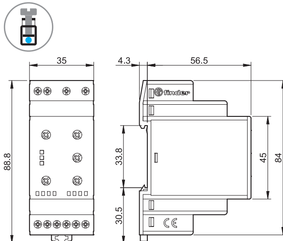
70.42 Винтовые клеммы
