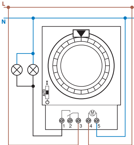
Тип 12.31
