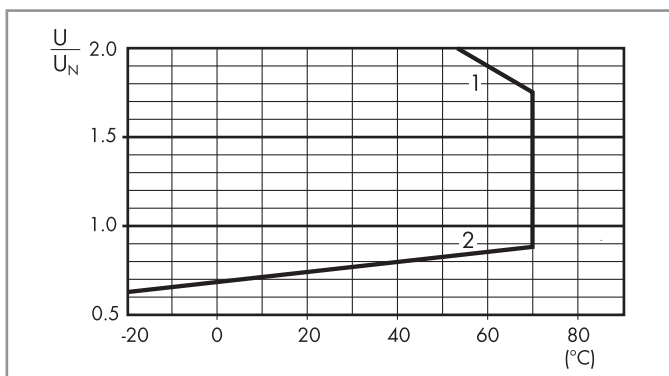
R 40 - Отношение рабочего диапазона для DC к температуре окр. среды - Чувствительная катушка, типы 40.11
