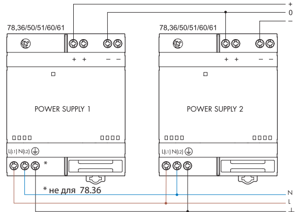
Соединение с двойной полярностью
