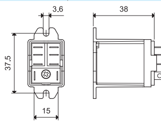
056.25 с реле
