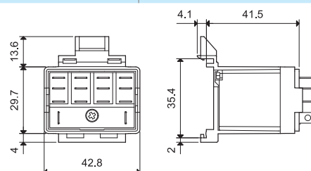
056.47 с реле
