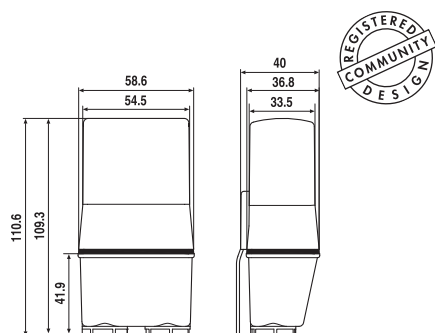
Тип 10.42
