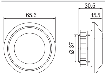
В упаковке – 2 клапана выравнивания давления
