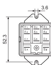
062.05 с реле
