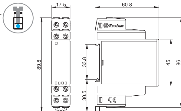
Тип 7P.37.8.275.1003
