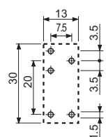
95.13.2 Вид сбоку
