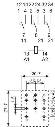
Вид со стороны выводов
