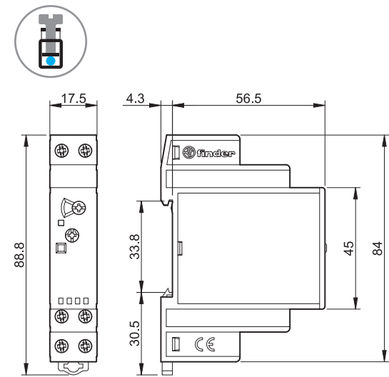
15.11 Винтовые клеммы
