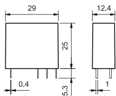
Тип 40.31/51/52/61 (страница 29)
