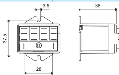
056.45 с реле
