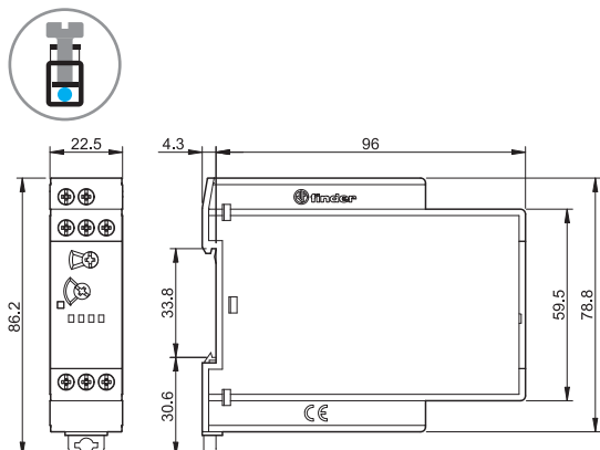
83.91 Винтовые клеммы
