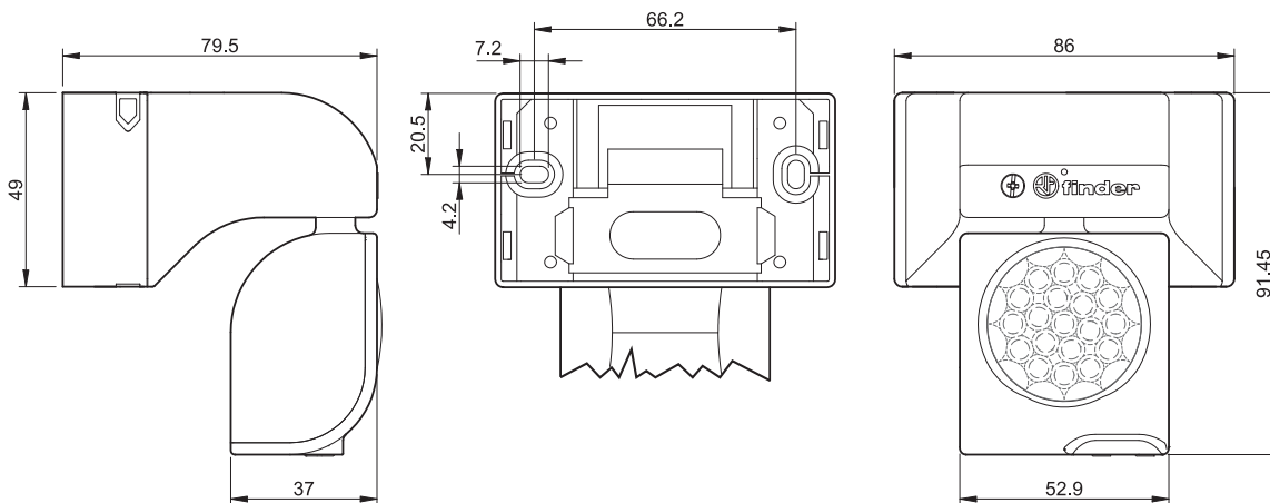
Тип 18.91
