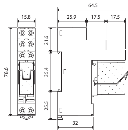
48.12 Винтовые клеммы
