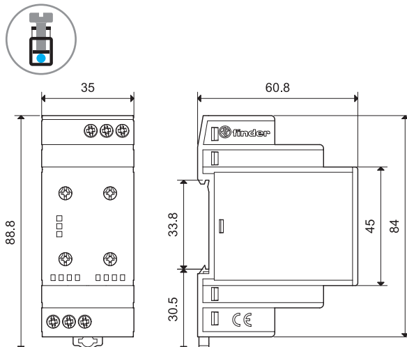
70.42 Винтовые клеммы
