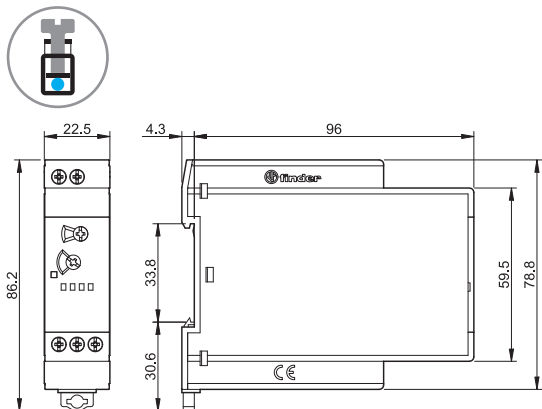
83.41 Винтовые клеммы
