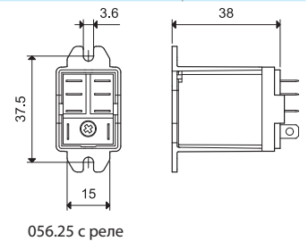
056.25 с реле
