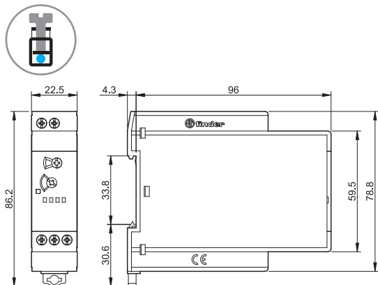
83.62 Винтовые клеммы
