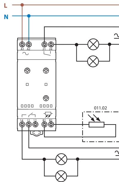
Тип 11.42
