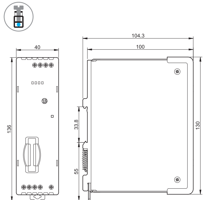
78.1B Винтовые клеммы
