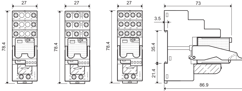
58.32 Винтовые клеммы
