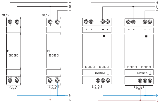
Соединение с двойной полярностью
