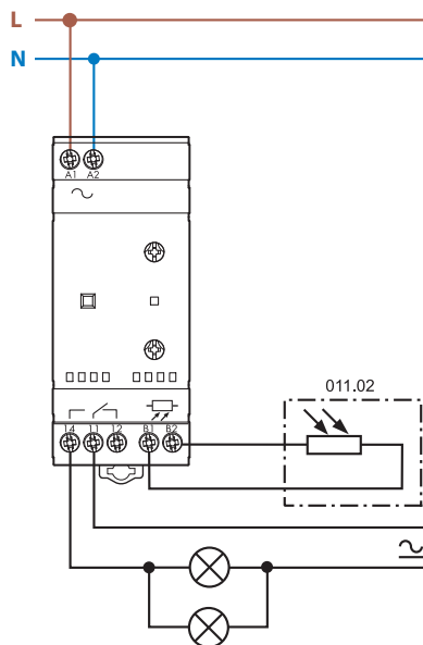
Тип 11.41
