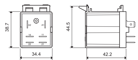
065.08 с реле
