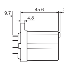
062.10 с реле
