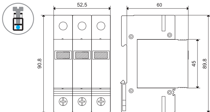
Тип 7P.23.9.000.6020
