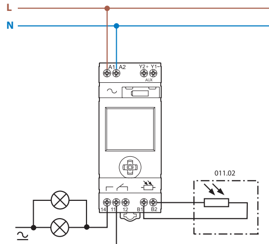
Тип 11.91
