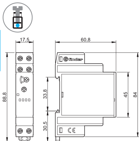
13.61 Винтовые клеммы
