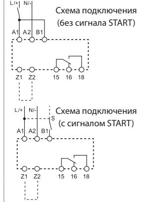
Схема подключения (без сигнала START)
