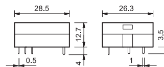
Тип 40.11 (страница 31)
