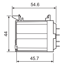
062.08 с реле
