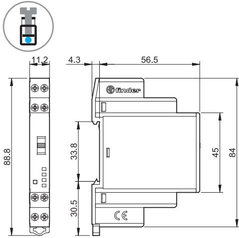
Тип 19.21
