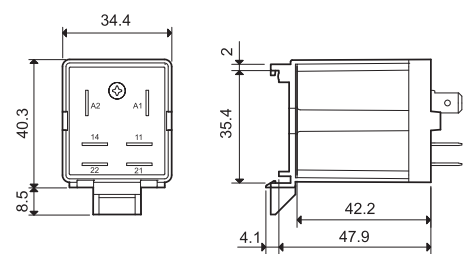
065.07 с реле
