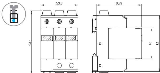
Тип 7P.26.9.000.1015
