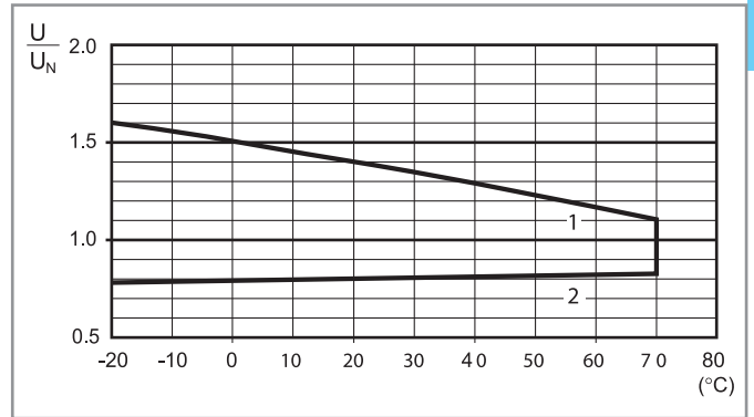
R 62 - Отношение рабочего диапазона для AC к температуре окр. среды - Переключающие контакты
