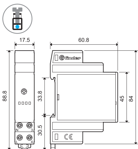
14.81 Винтовые клеммы
