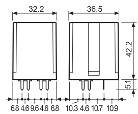
Тип 65.61- 0300
